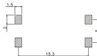
安装图 instructions
