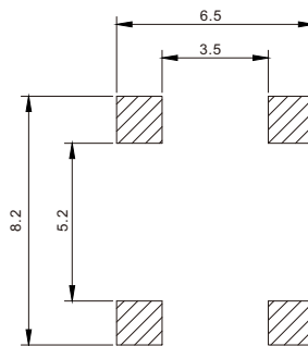
安装图
